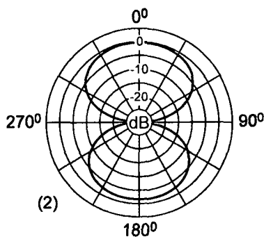
דו כיווני
