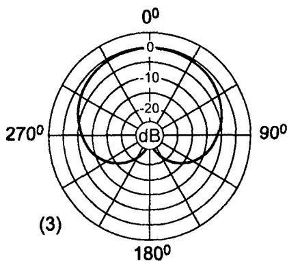
חד כיווני
